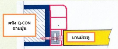
การติดตั้งแบบแห้ง
